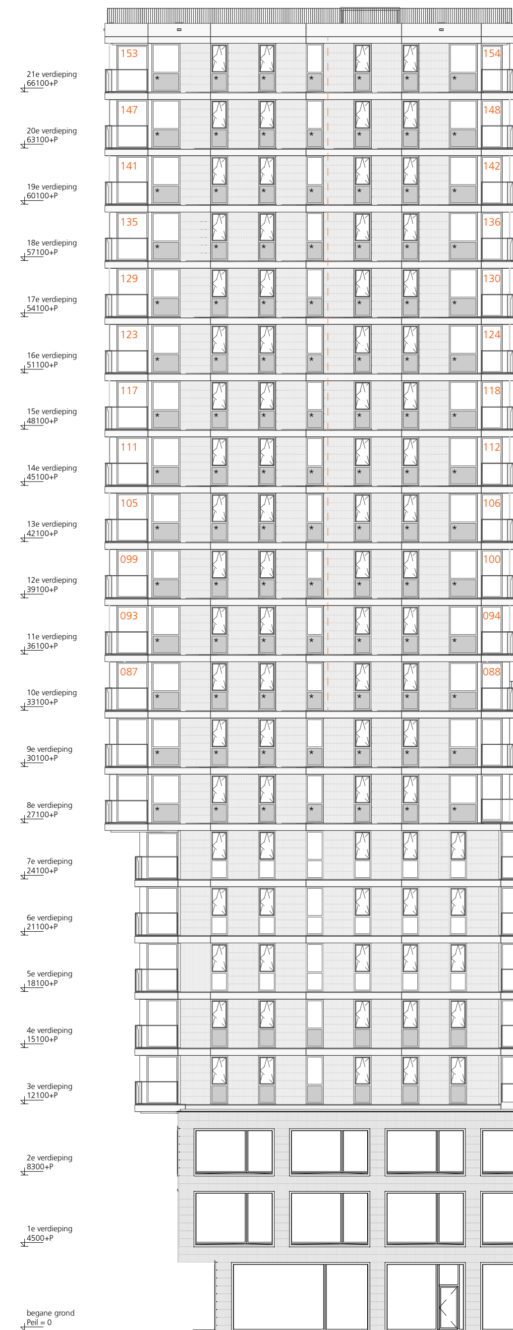
gebouw 1
