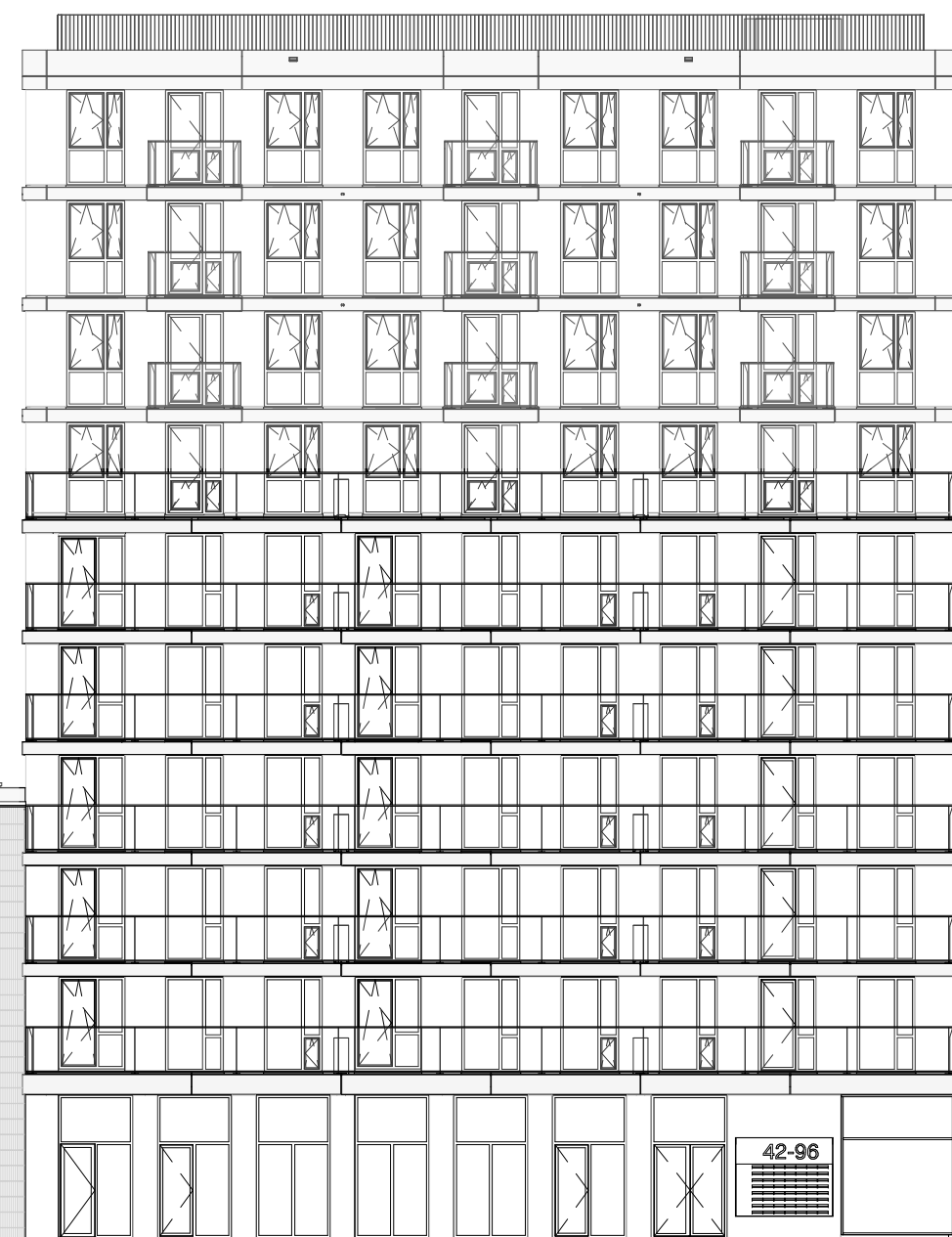
gebouw 2 - huurwoningen
